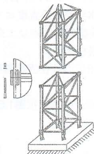
图1.5.1-2 吊装标准节
