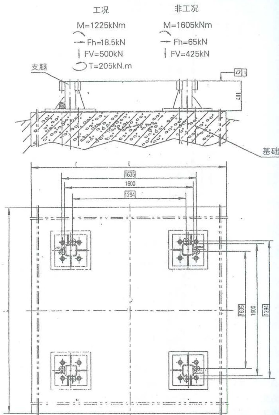
附 1: 采用短支腿固定方式示意图
