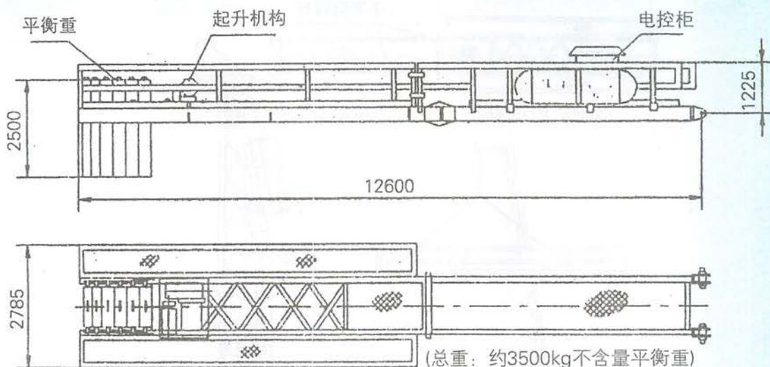
图1.5.6-1 平衡臂总成
