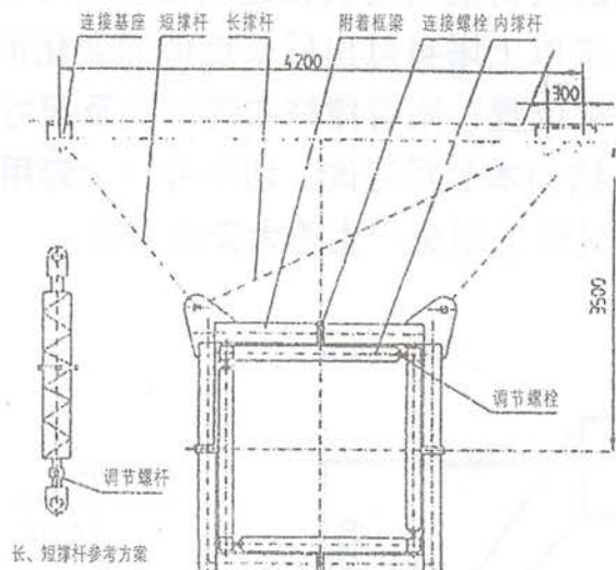
图1.9-1B附着架示意图
