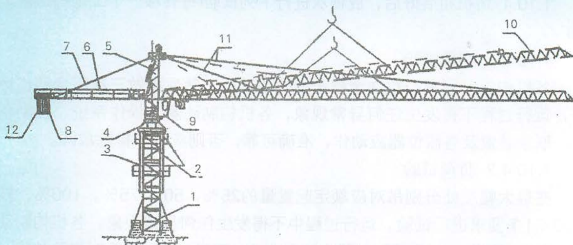
图1.10-2 底架固定式塔机安装顺序示意图
