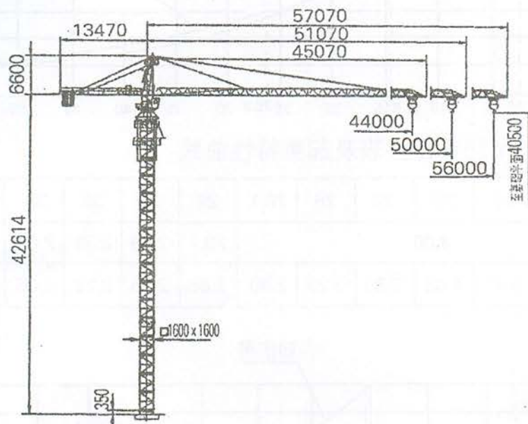
图1 QTZ63-1塔式起重机支腿固定独立式外形尺寸
