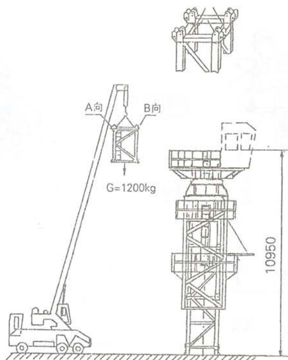
图1.5.4-2 吊回转塔身
