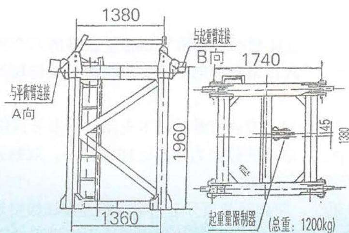
图1.5.4-1 回转塔身
