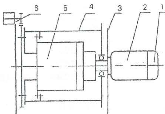
1.电磁盘式制动器 2.电动机 3.支架 4.卷筒 5.减速器 6.限位器
