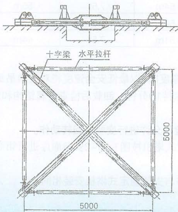
图1.10-3 底架组装
