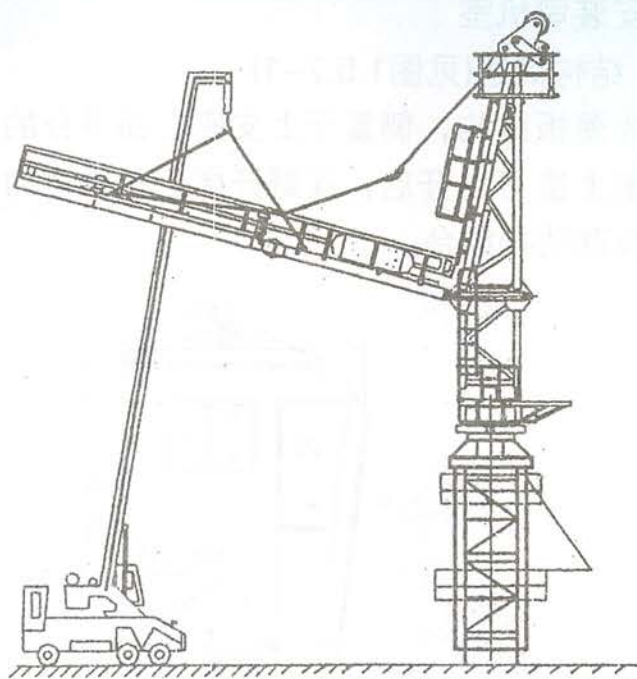
图1.5.6-4 安装平衡臂拉杆
