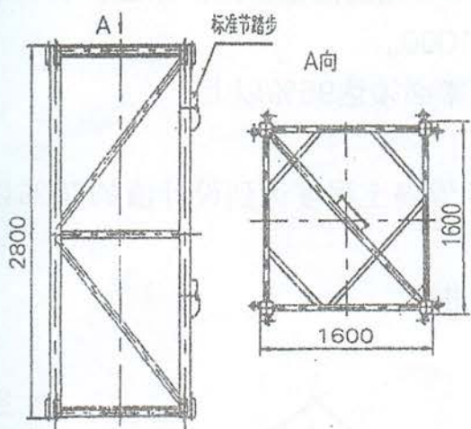
图1.5.1-1 标准节
