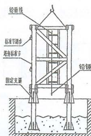
图1.4-4 固定支腿的浇注示意图
