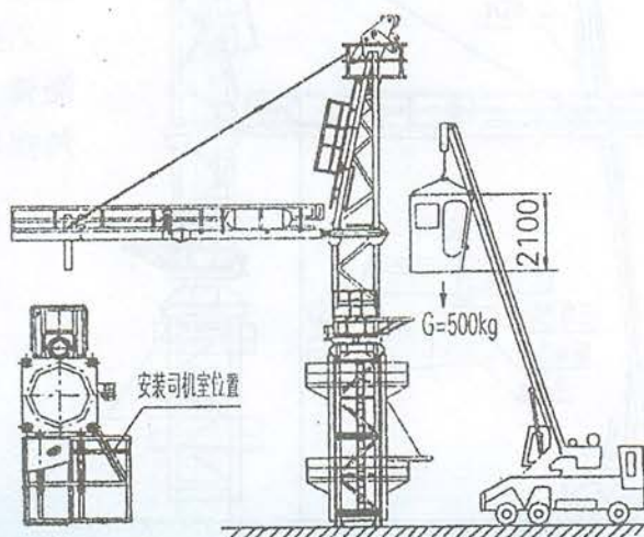
图1.5.7-2 吊装司机室
