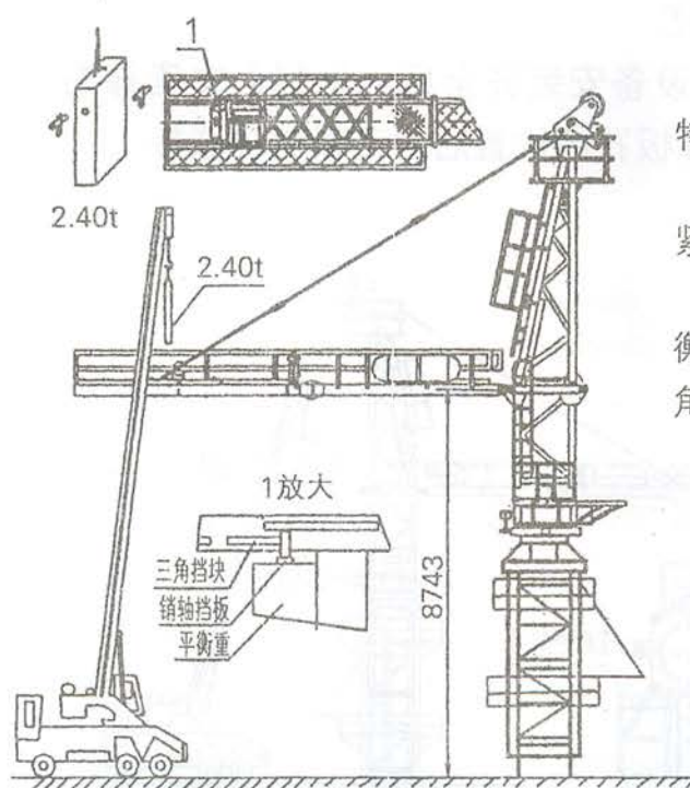
图1.5.6-5 安装一块平衡重
