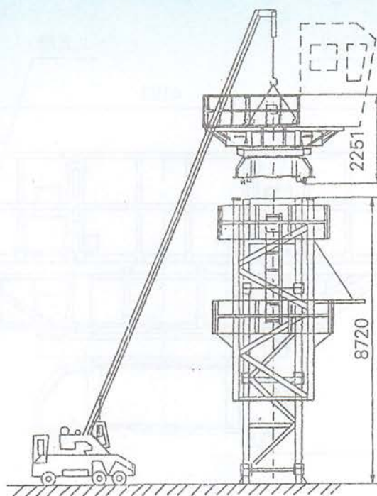
图1.5.3-2 吊回转总成
