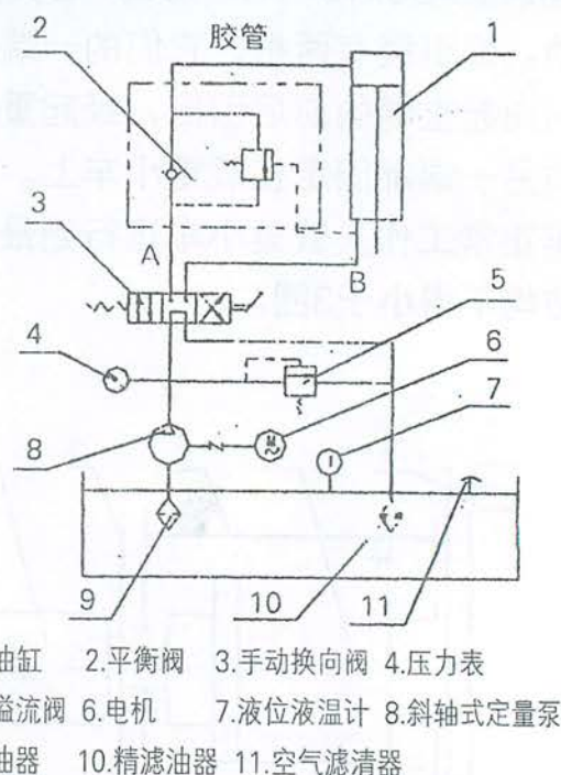
图2.2-6 液压系统图
