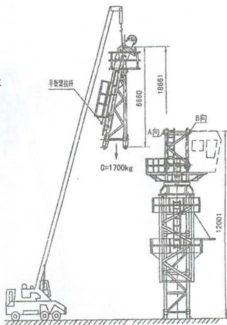
图1.5.5-2 吊装塔顶
