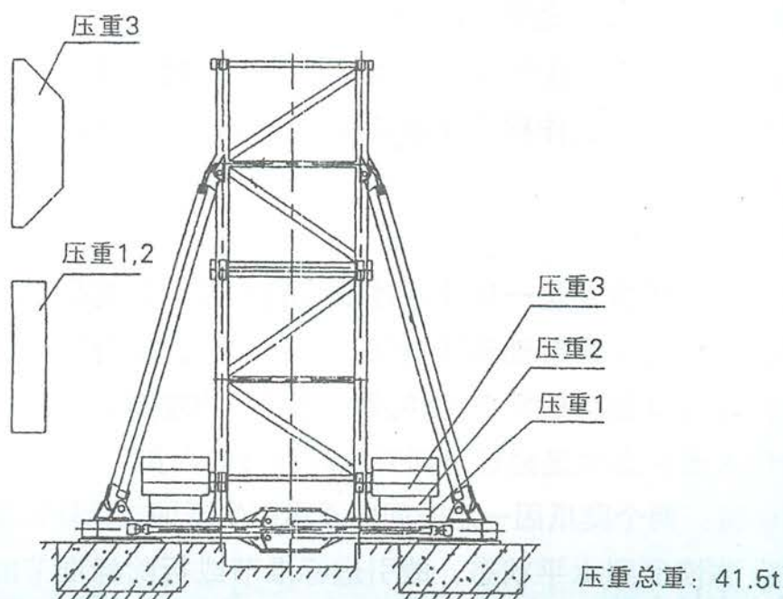
图1.10-5 压重安装
