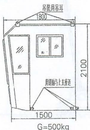
图1.5.7-1 司机室
