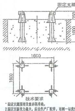
图1.4-3 固定支腿固定方式示意图
