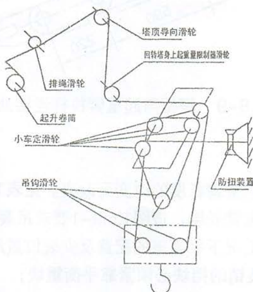
图1.6-1 起升钢丝绳绕绳示意图
