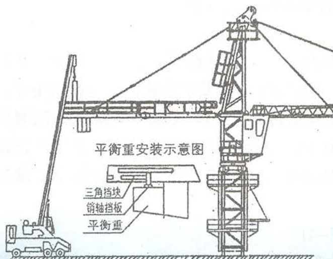
图1.5.9-1 吊装平衡臂
