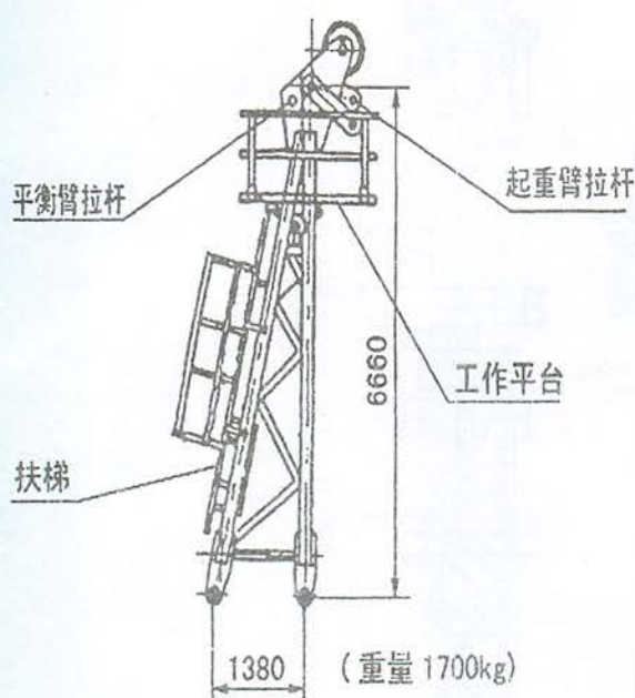
图1.5.5-1 塔顶
