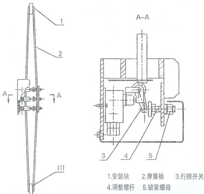
3.2-1 力矩限制器示意图
