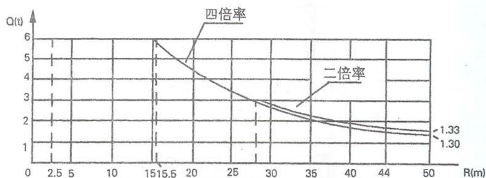
9.3.3 44m起重特性表及起重特性曲线
