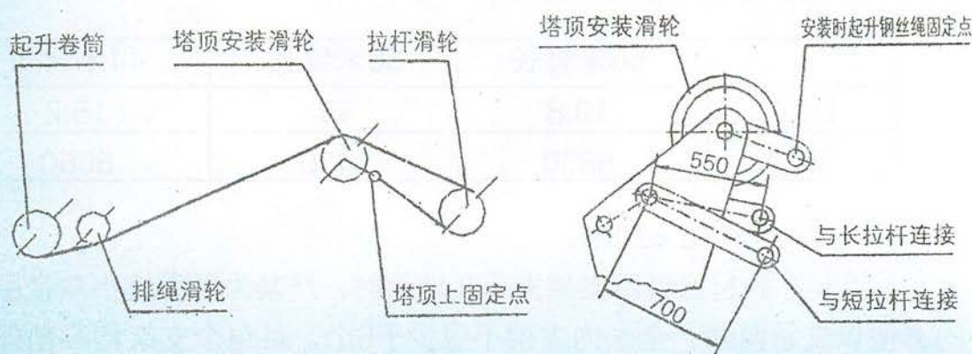
图1.5.8-7 安装起重臂拉杆时起升钢丝绳绕法 图1.5.8-8与起重臂拉杆连接处塔帽结构
