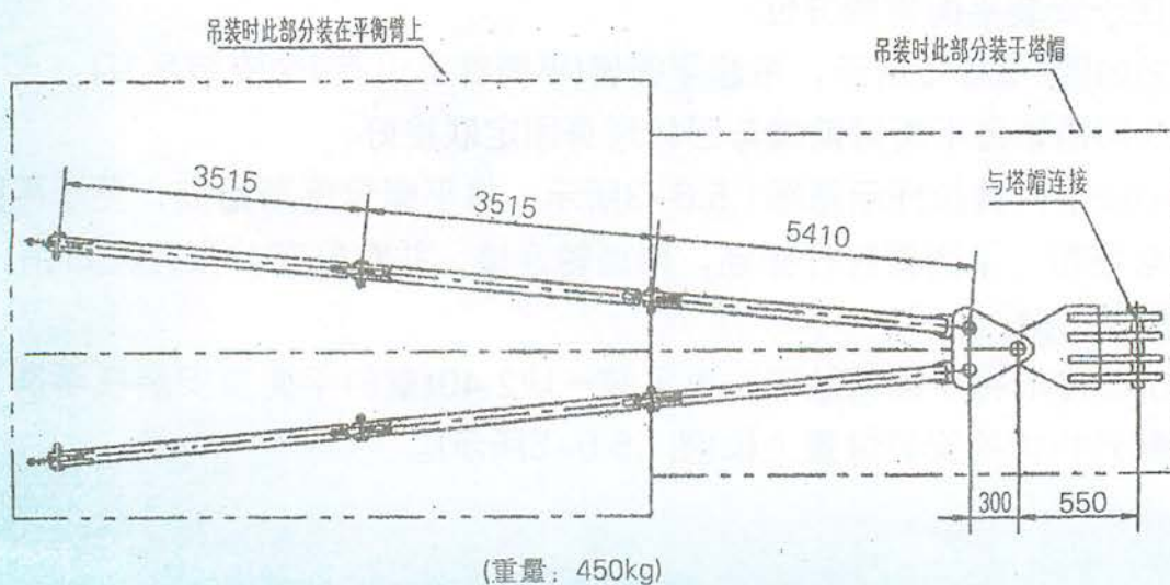
图1.5.6-3 平衡臂拉杆总成
