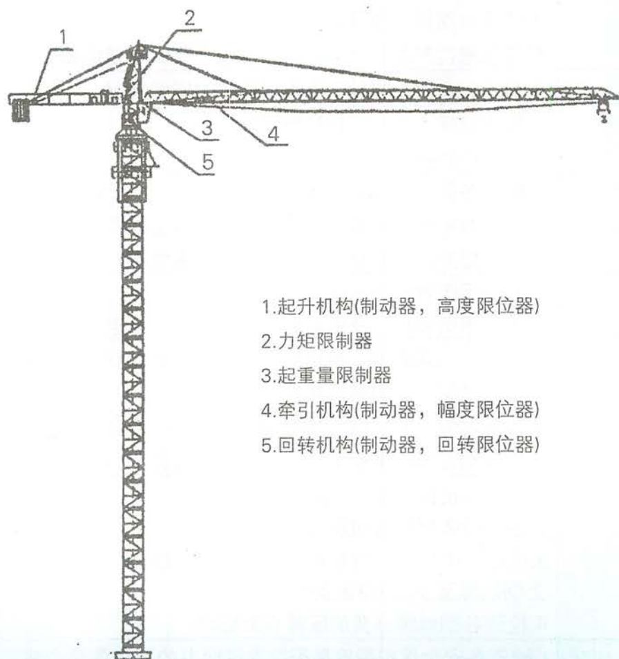
图1.10-1 整机安全保护装置的安装位置
