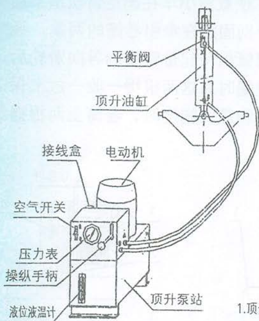
图2.2-5 顶升系统液压管示意图
