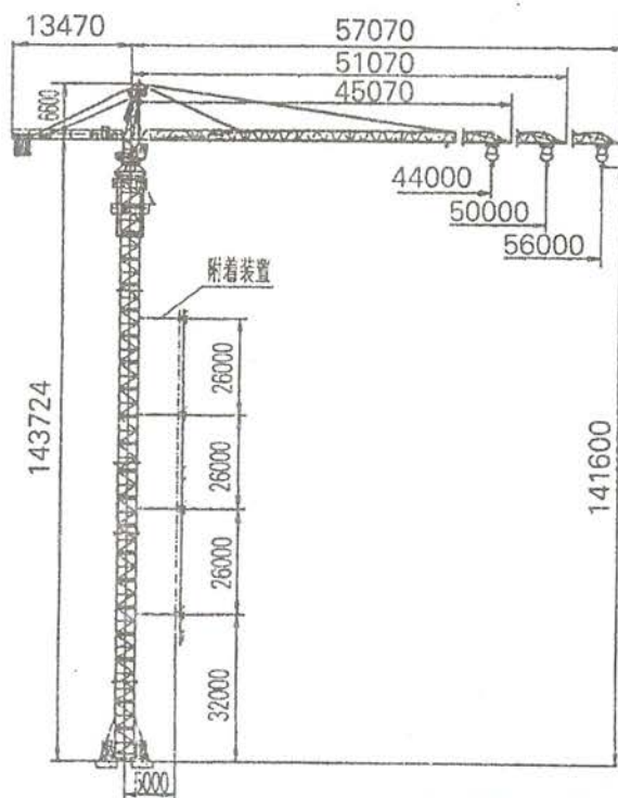
图4 QTZ63-1塔式起重机底架固定附着式外形尺寸
