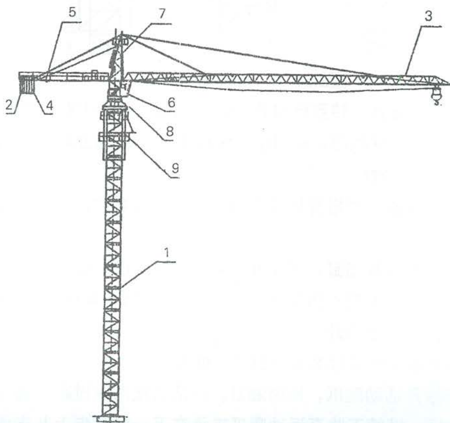
图2.2-1 塔式超重机拆卸。
