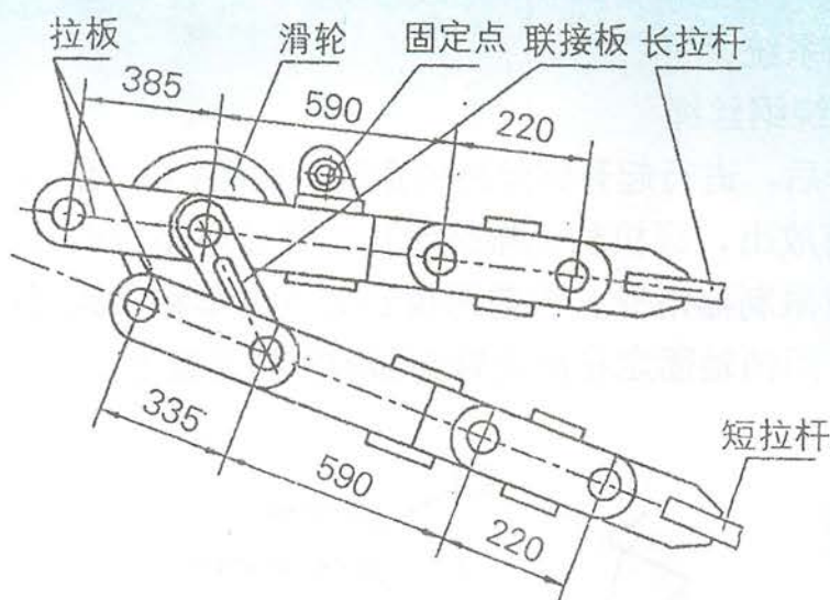
图1.5.8-9 塔帽与起重臂拉杆连接处结构
