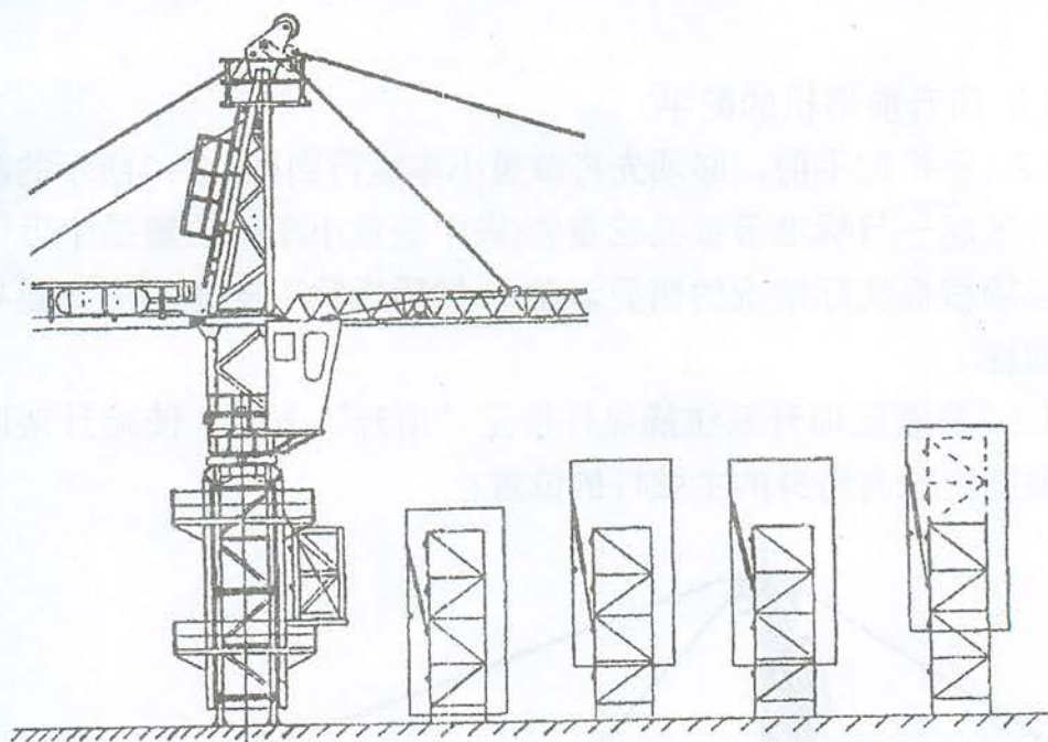
图1.8-2 顶升过程
