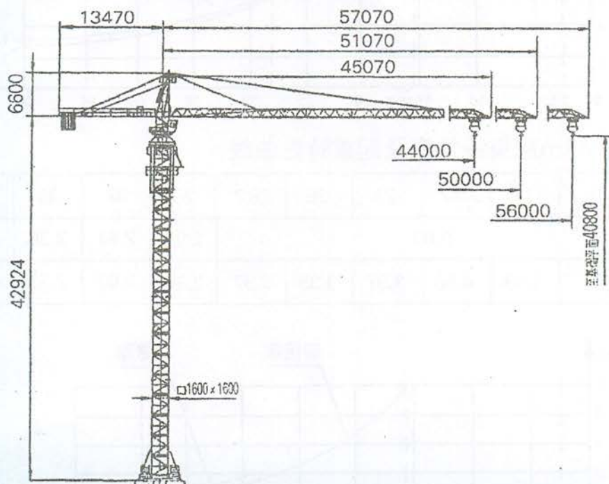
图2 QTZ63-1塔式起重机底架固定独立式外形尺寸
