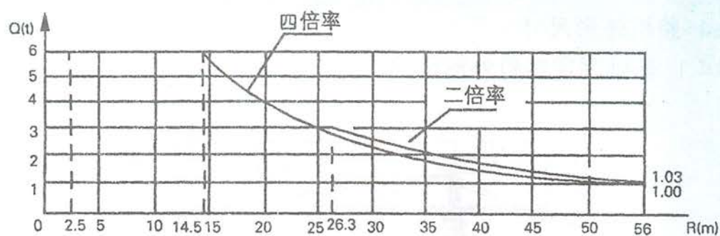
9.3.2 50m起重特性表及起重特性曲线
