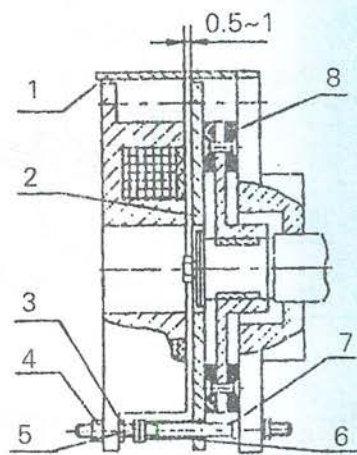
1.制动器罩 2.衔铁 3,4,5调整螺母 6.制动弹簧 7.导向螺栓 8.摩擦片
