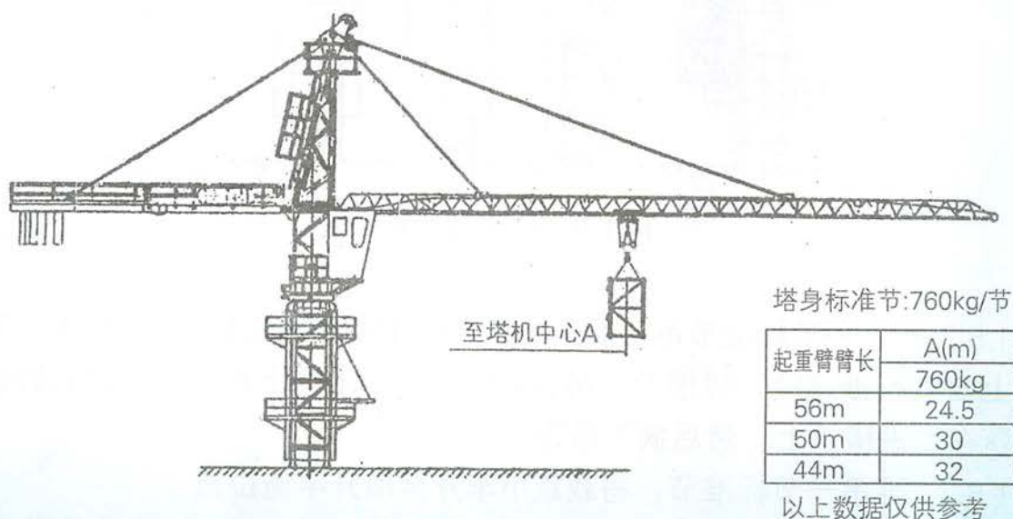
图1.8-1 顶升前的平衡
