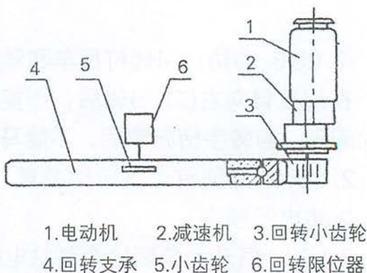
图2.2-2 回转机构传动系统图
