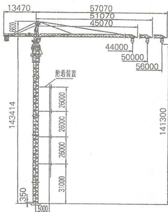
图3 QTZ63-1塔式起重机支腿固定附着式外形尺寸
