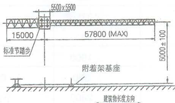
图1.2-1 塔机安装场地的参考尺寸
