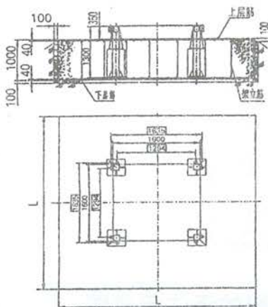
图1.4-2 固定基础
