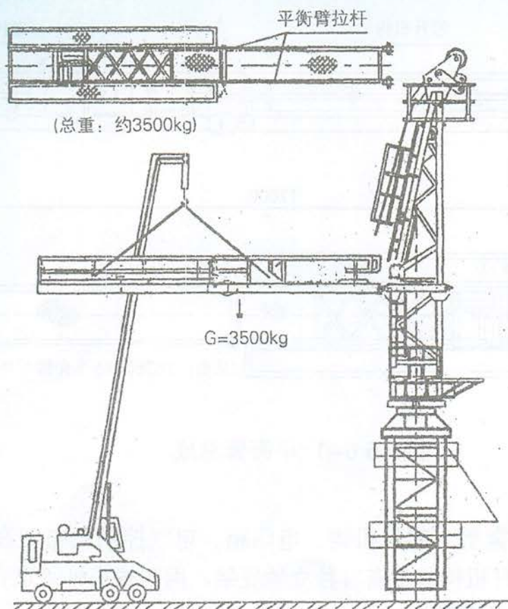
图1.5.6-2 吊平衡臂
