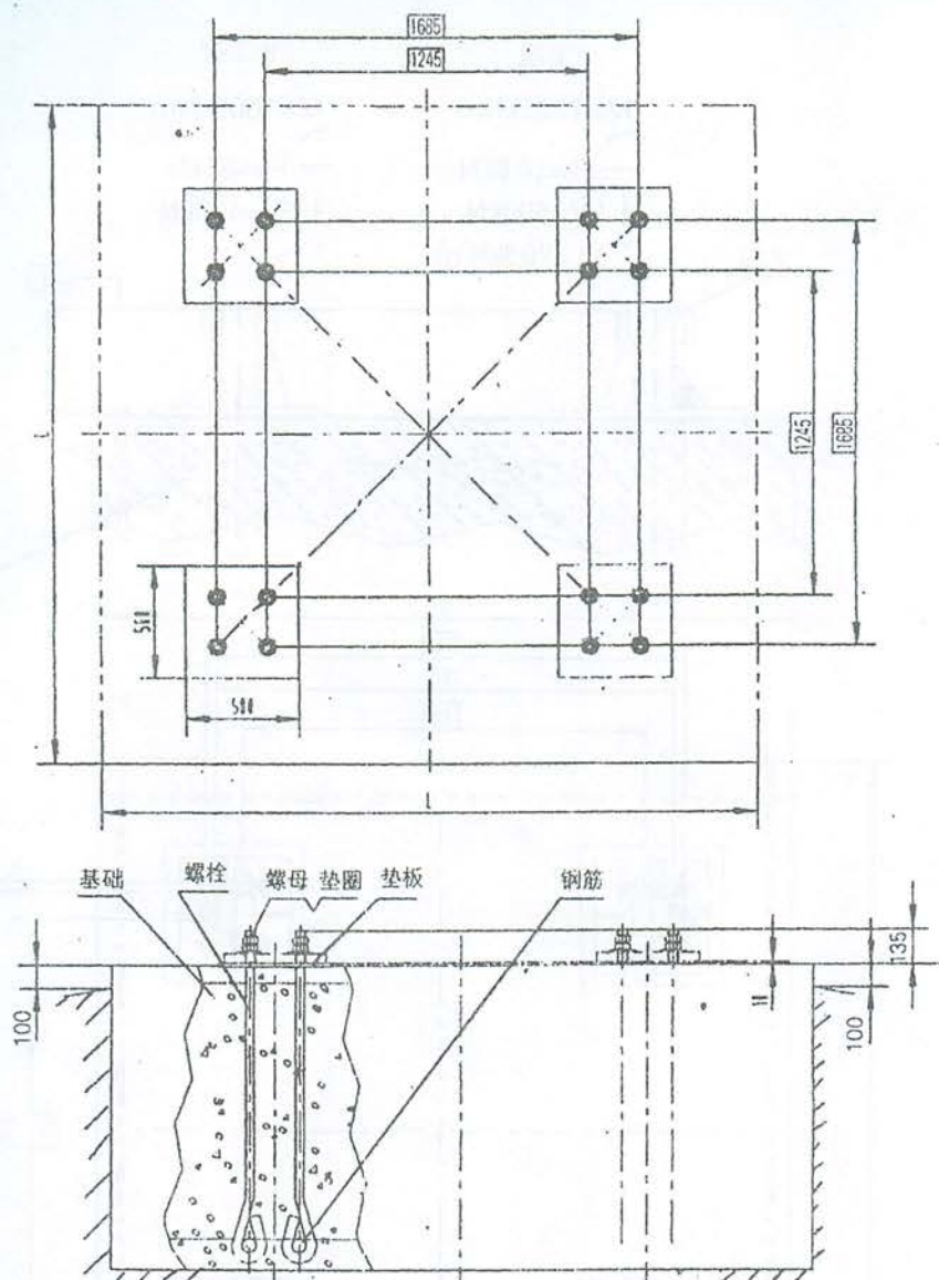
附2：短支腿固定方式地脚螺栓安装示意图
