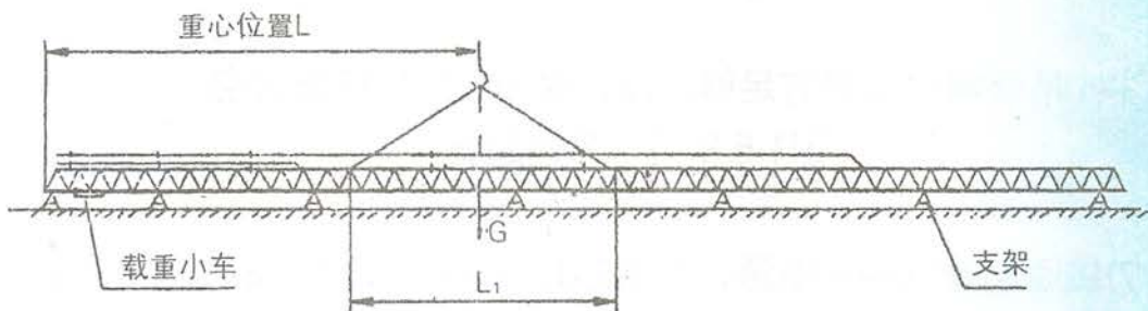
图1.5.8-5 起重臂重心
