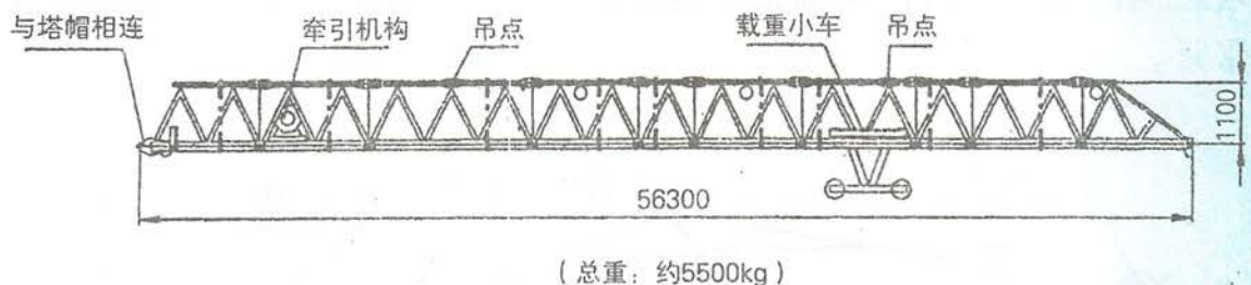
图1.5.8-1起重臂结构
