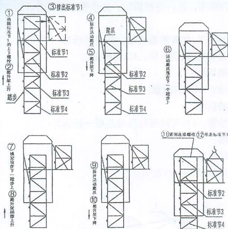
图2.2.1-1 拆卸塔身
