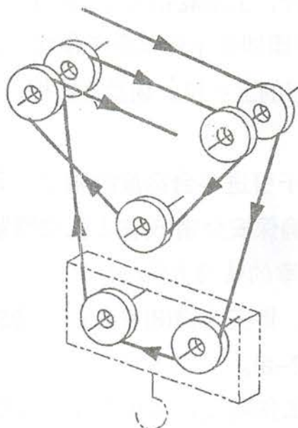
图1.7-2 起升钢丝绳在载重小车总成上绕绳示意图
