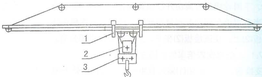
1. 载重小车 2. 上滑轮组 3. 下滑轮组
