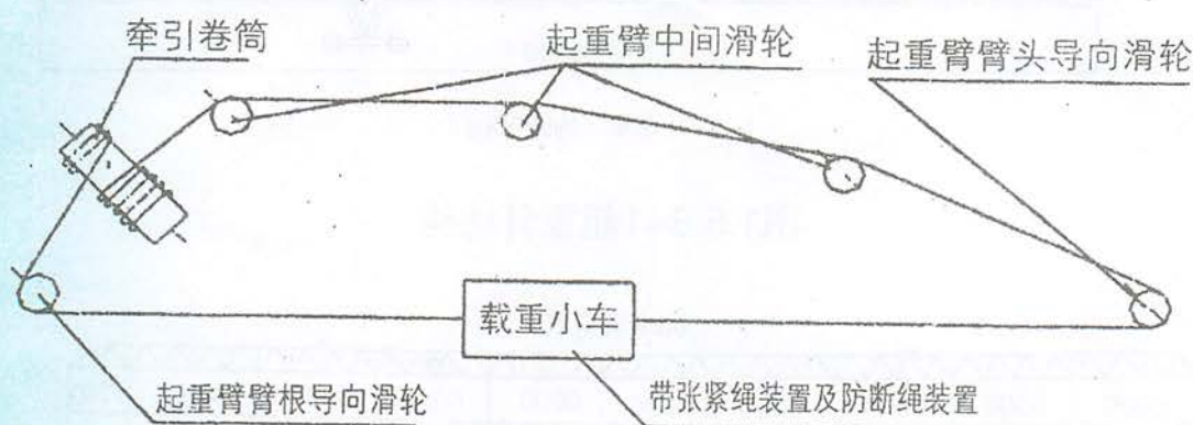
图1.5.8-3 牵引钢丝绳绕绳示意图
