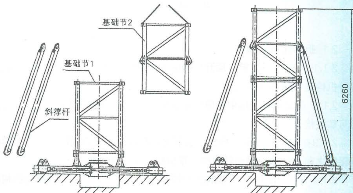
图1.10-4 底架基础节及斜撑杆的组装
