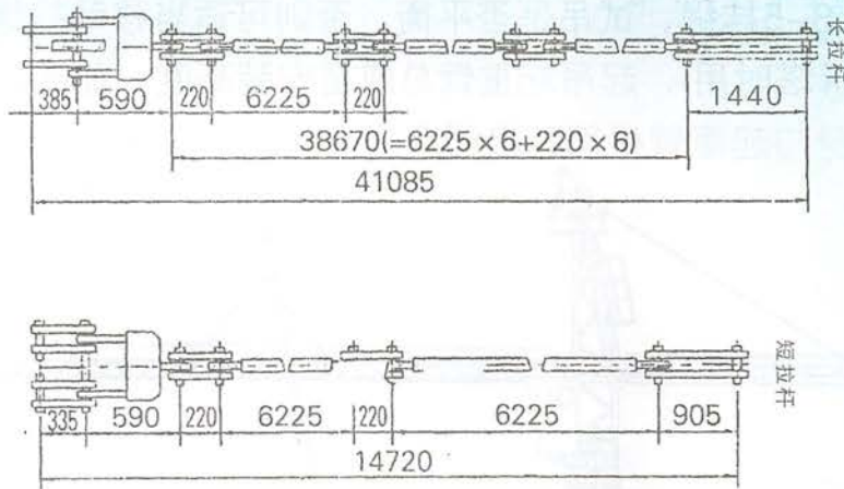
图1.5.8-4 牵引钢丝绳绕绳示意图
