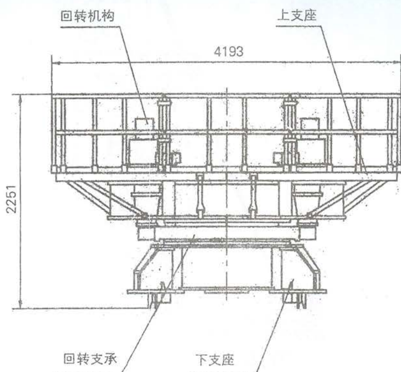
图1.5.3-1 回转总成
