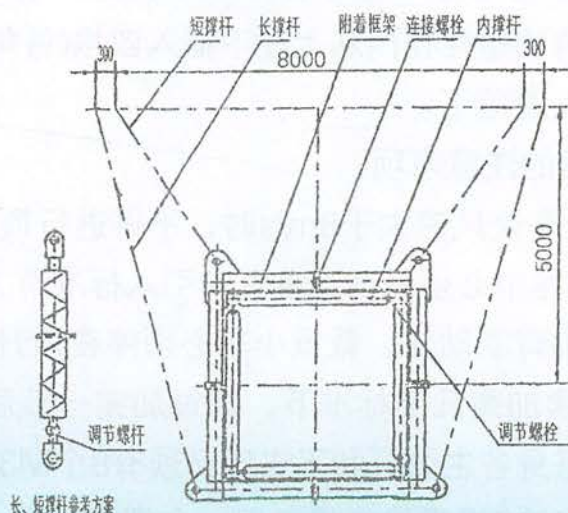
图1.9-1A 附着架示意图
