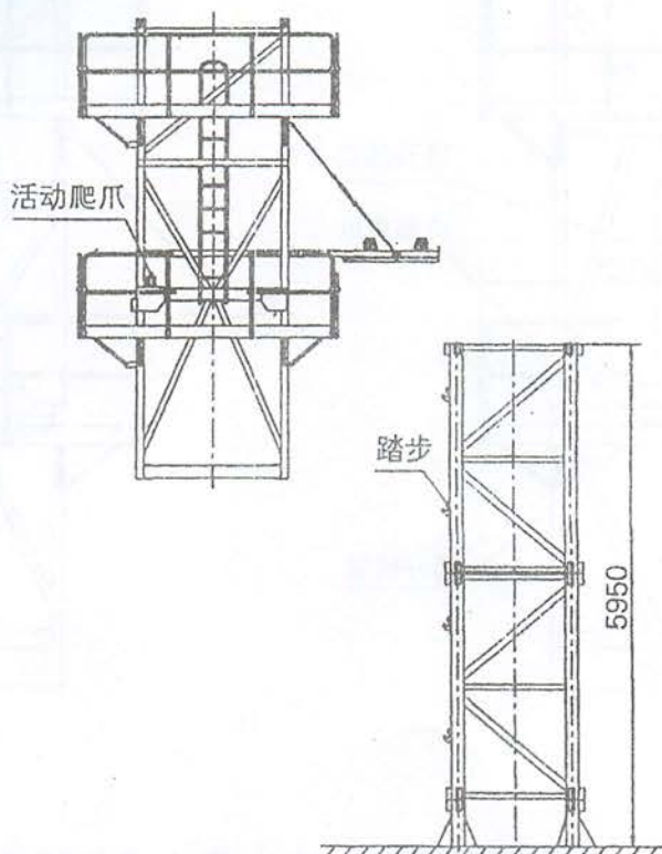
图1.5.2-2 吊装爬升架
