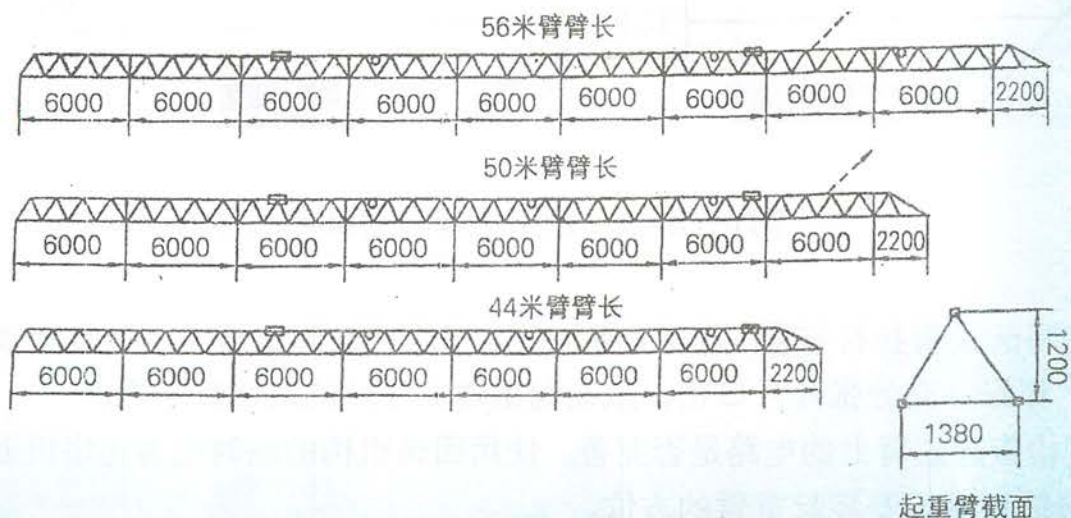
图1.5.8-2起重臂的组装
